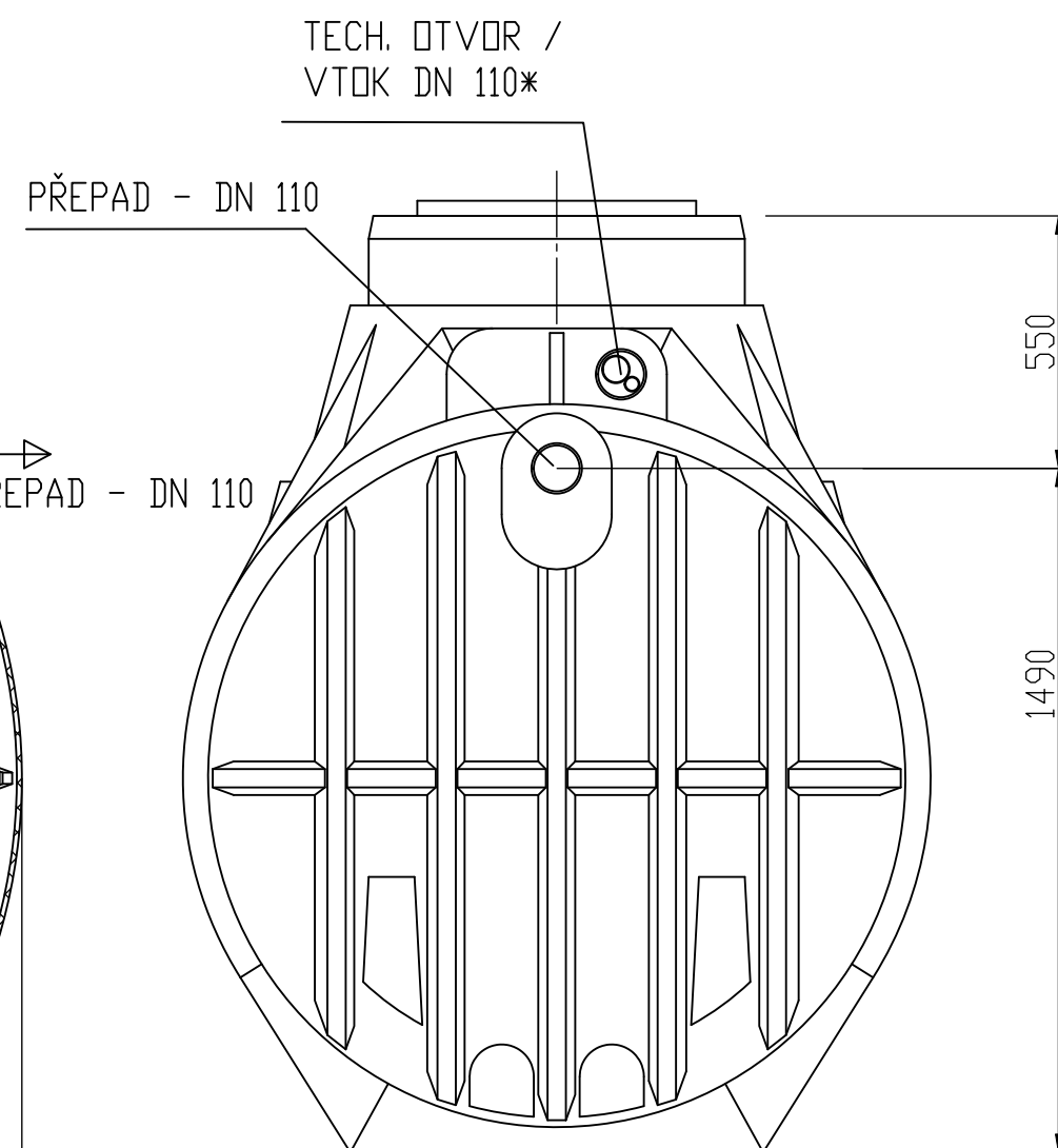
BOČNÍ POHLED 2
