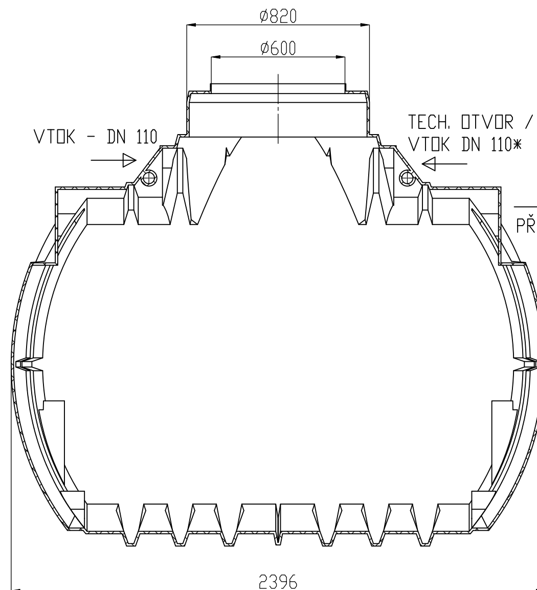
PODÉLNÝ ŘEZ A-A
