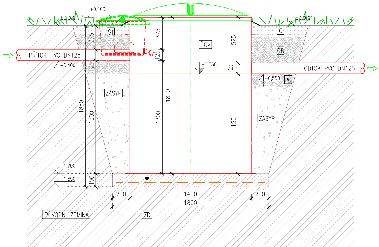
ŘEZ - OSAZENÍ
