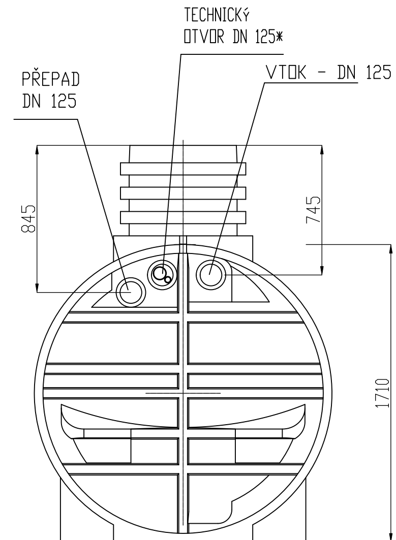
BOČNÍ POHLED 2
