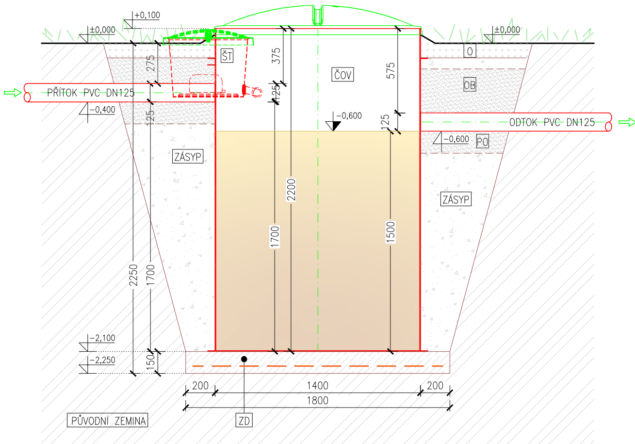
ŘEZ - OSAZENÍ
