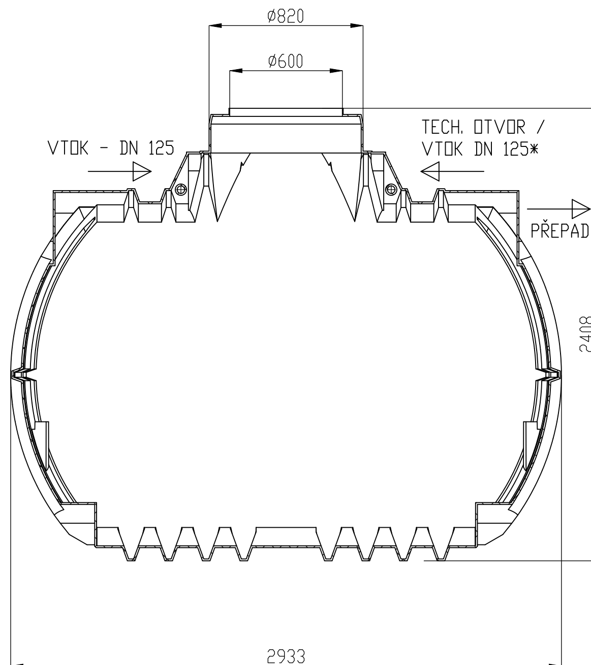
PŘEPAD - DN 125
