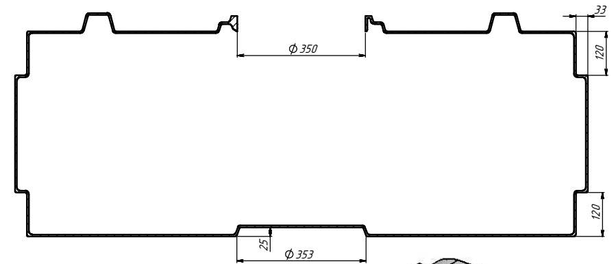
СЕЧЕНИЕ А-А
