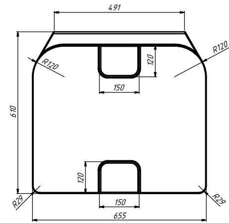
СЕЧЕНИЕ А-А
